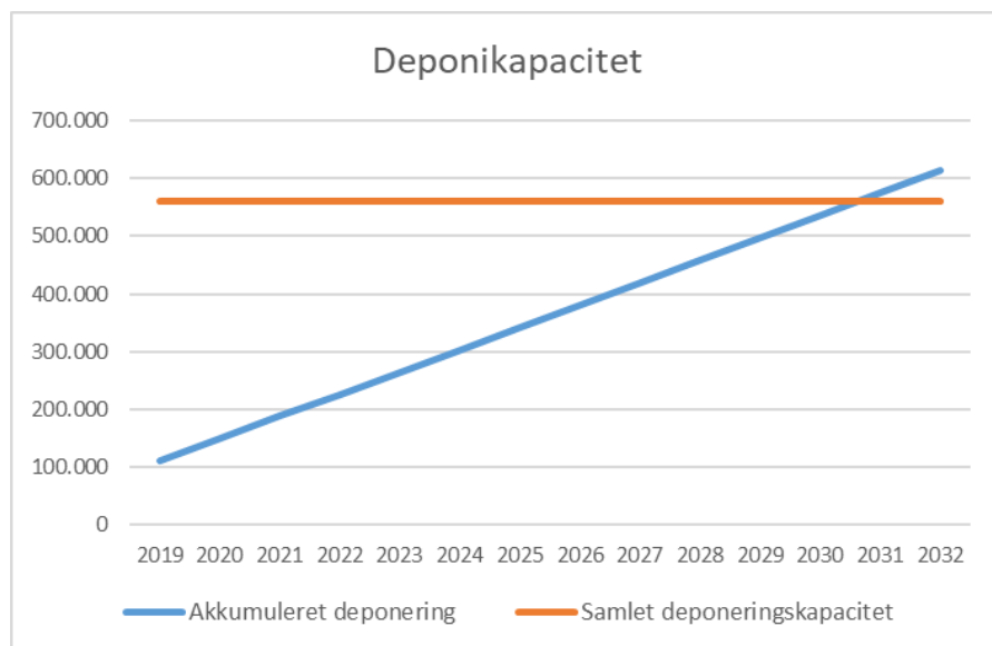
Figur 6: Akkumulerede affaldsmængder til deponi og deponeringskapacitet
