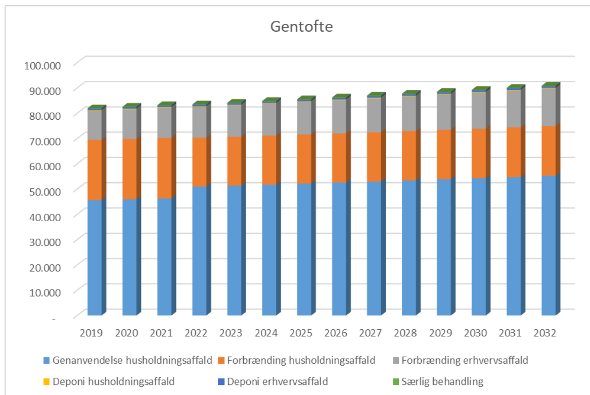
Figur 2: Fremskrivning af Gentofte Kommunes husholdnings- og erhvervsaffald fordelt på behandlingsform
