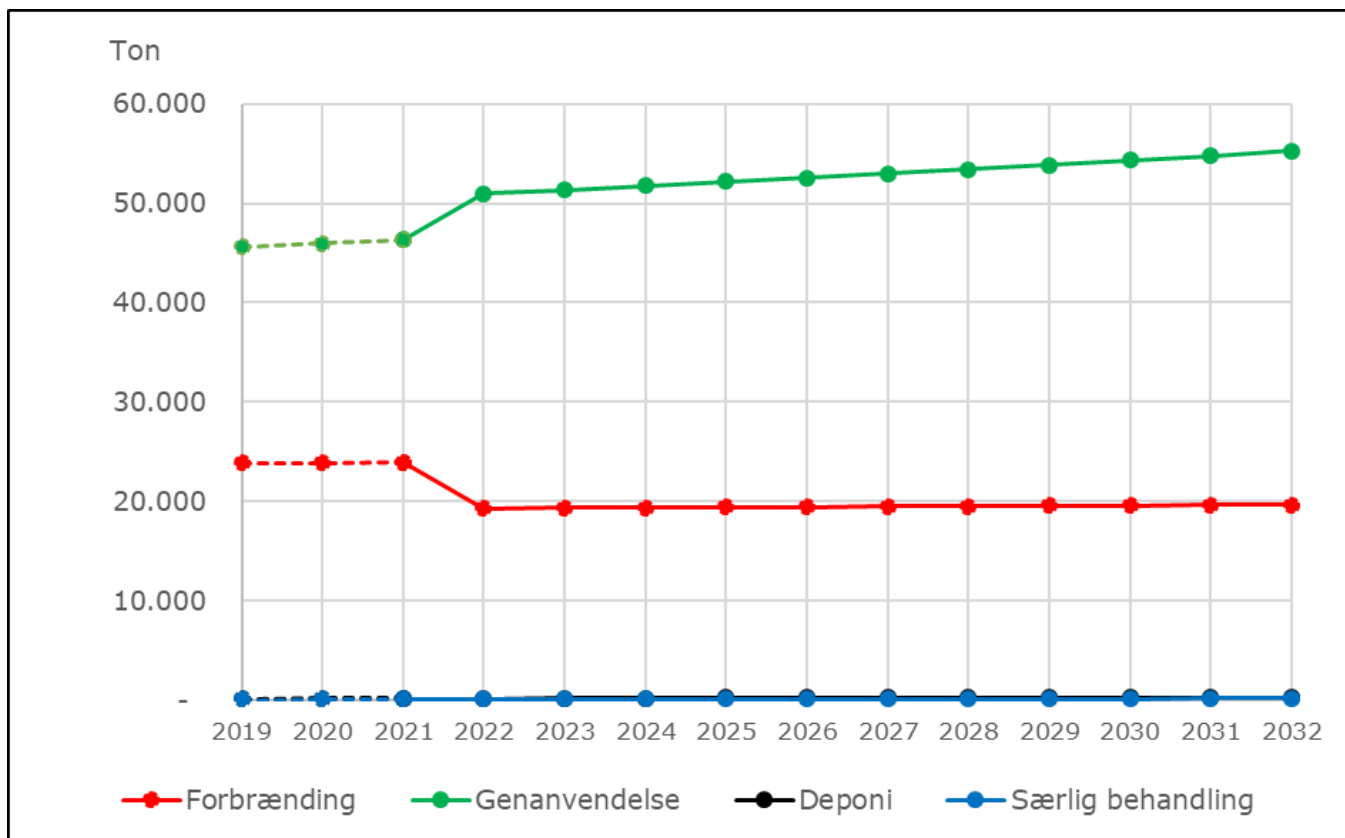
Figur 1: Fremskrivning af Gentofte Kommunes husholdningsaffald fordelt på behandlingsform ved særskilt indsamling af 10 affaldsfraktioner.
