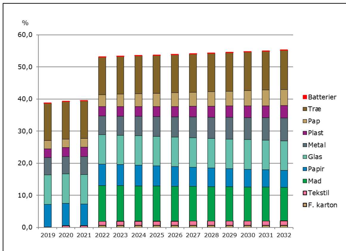
Figur 3: Forventede genanvendelsesprocenter i Gentofte Kommune ved særskilt indsamling og sortering af 10 fraktioner.
